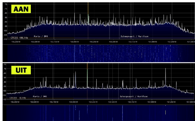
PV-Installatie bij de directe burens aan (boven) en uit (onder). Het verschil is heel duidelijk te zien.
